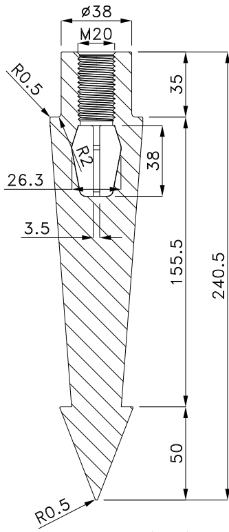
SECTION A-A
